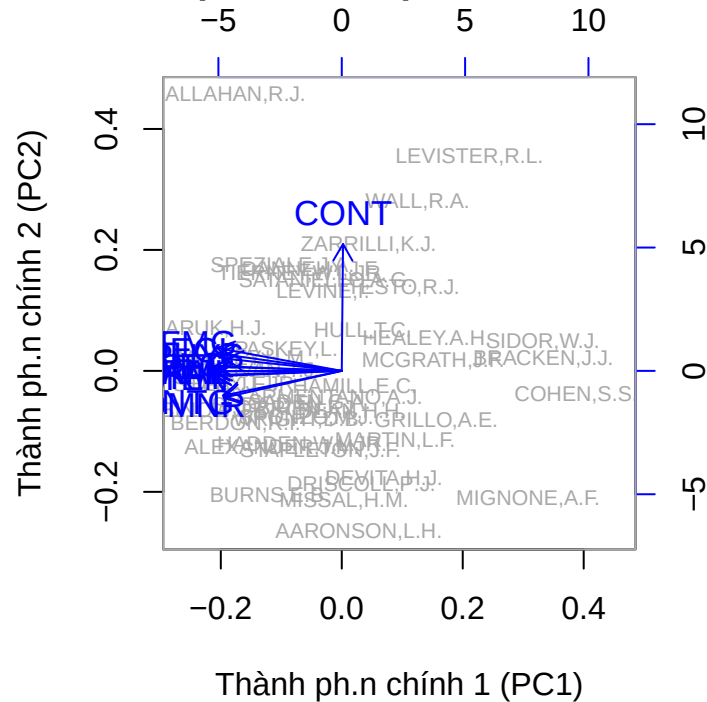
Biểu đồ hai thành phần chính (dựa trên ma trận tương quan)
