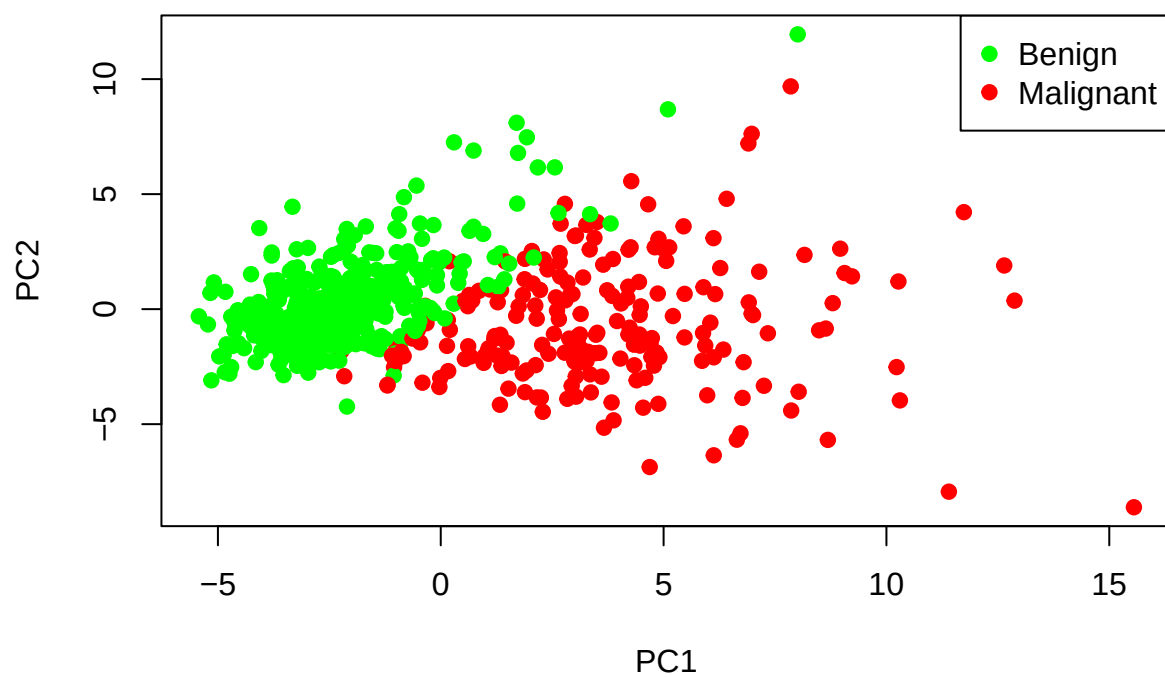
Bi.u d. phân tán PC1 và PC2 (Màu theo Diagnosis)
